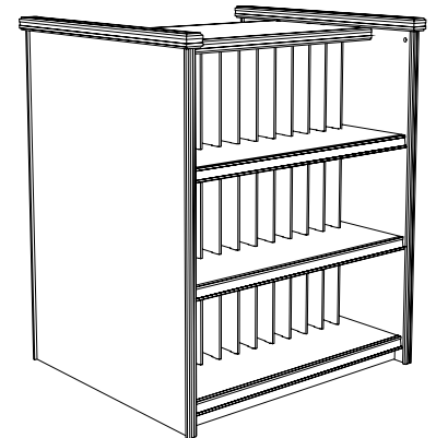
L. 3-level Gondola w/Dividers
